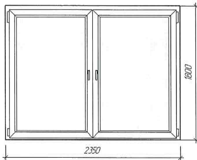
Схема существующих окон
