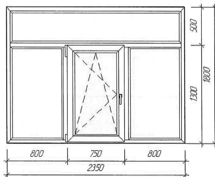
Схема планируемых к установке окон ПВХ
